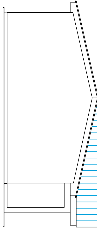
PIGNON GAUCHE
